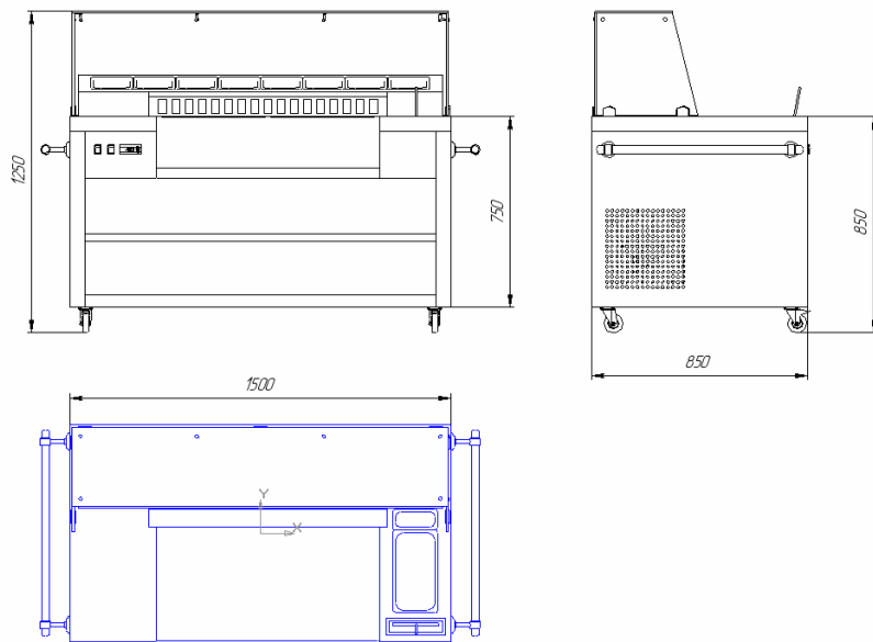
Рис. 1 Блинная станция с охлаждаемой ванной
