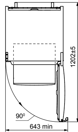
Şəkil 2 – Soyuducu (yuxarıdan görüntüsü)
