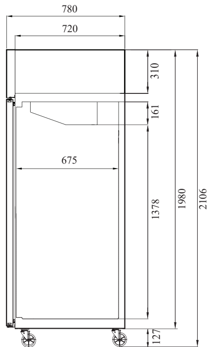
ВИД СБОКУ
