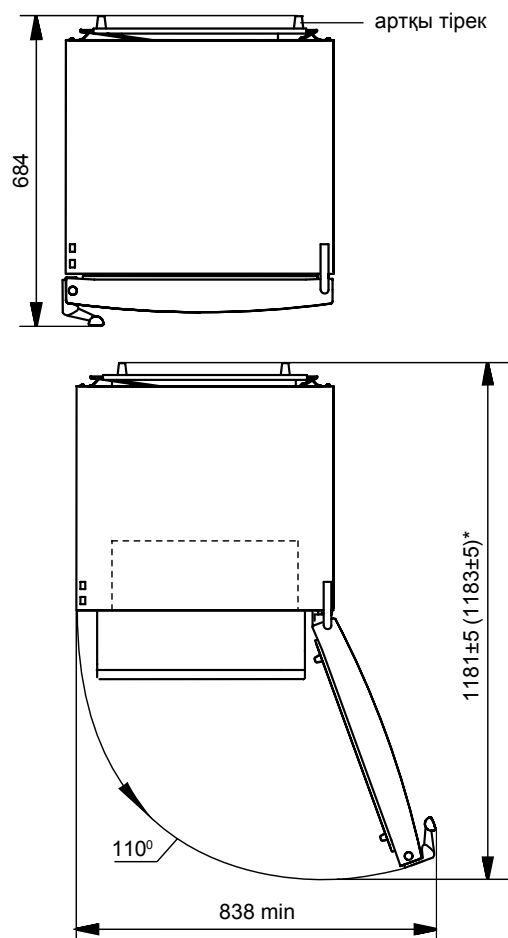
2-сурет – Тоңазытқыш (жоғарыдан қарағанда)
