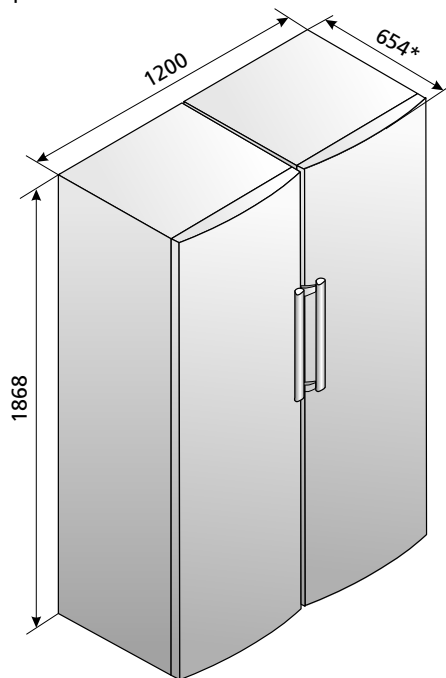
9-сурет – Side by side комбинациясының габариттік өлшемдері
