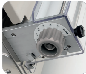
Manopole regolazione spessore rulli in alluminio Adjustable thickness by aluminium knobs
