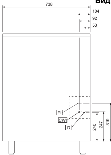
Вид спереди
