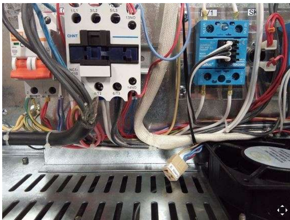
Рис.2 Место подключения шнура питания зонта к колодке 45 7373 9005 пароконвектомата
