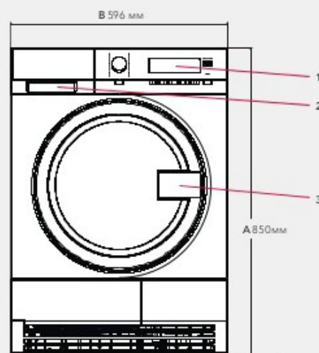
Передняя часть
