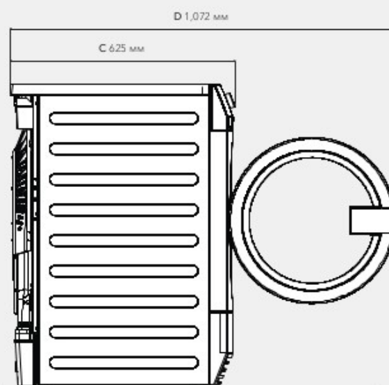
Правая сторона
