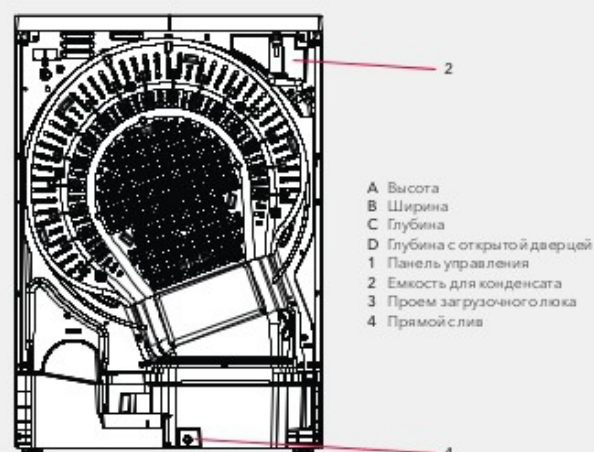
Задняя сторона
