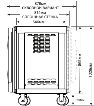
ВИД СБОКУ: ДВОЙНАЯ ГНУТАЯ ДВЕРЬ, СПЛОШНАЯ ЗАДНЯЯ СТЕНКА
