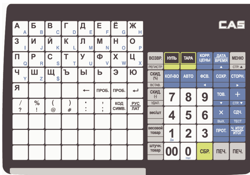
Рисунок 1.9 – Вид клавиатуры весов модификации CL3000-P
