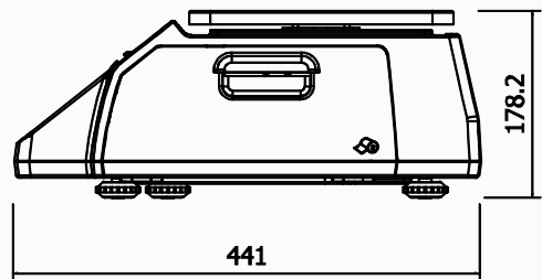
Рисунок 1.2 – Вид весов CL3000-B в геометрической проекции
