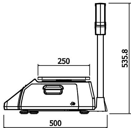
Рисунок 1.3 – Вид весов CL3000-P в геометрической проекции
