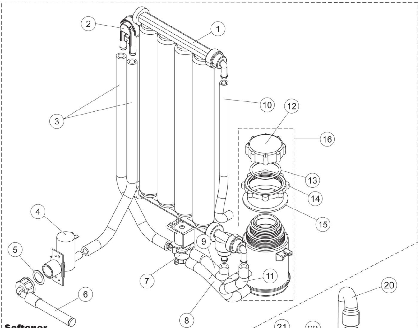
Softener Addolcitore
