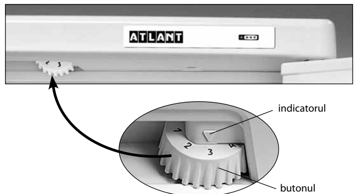
Figura 3 — Reglarea temperaturii
