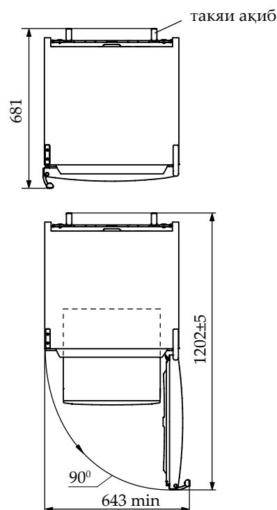
Расми 2 – Яхдон (намои болоӣ)
