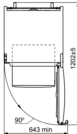
2-сүрөт – Муздаткыч (үстүнөн караганда)
