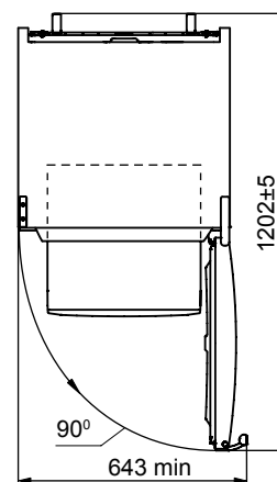
2-расм – Совуткич (юқоридан кўриниши)
