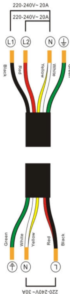
Схема подключения кабелей
