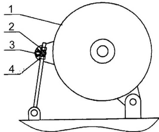
Схема №20 Регулировка натяжения ремней.
