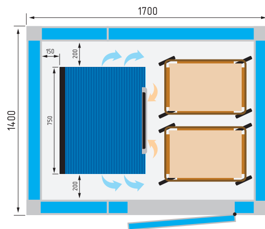
BCF 40.1.T2; BCF 40.1.T2inox
