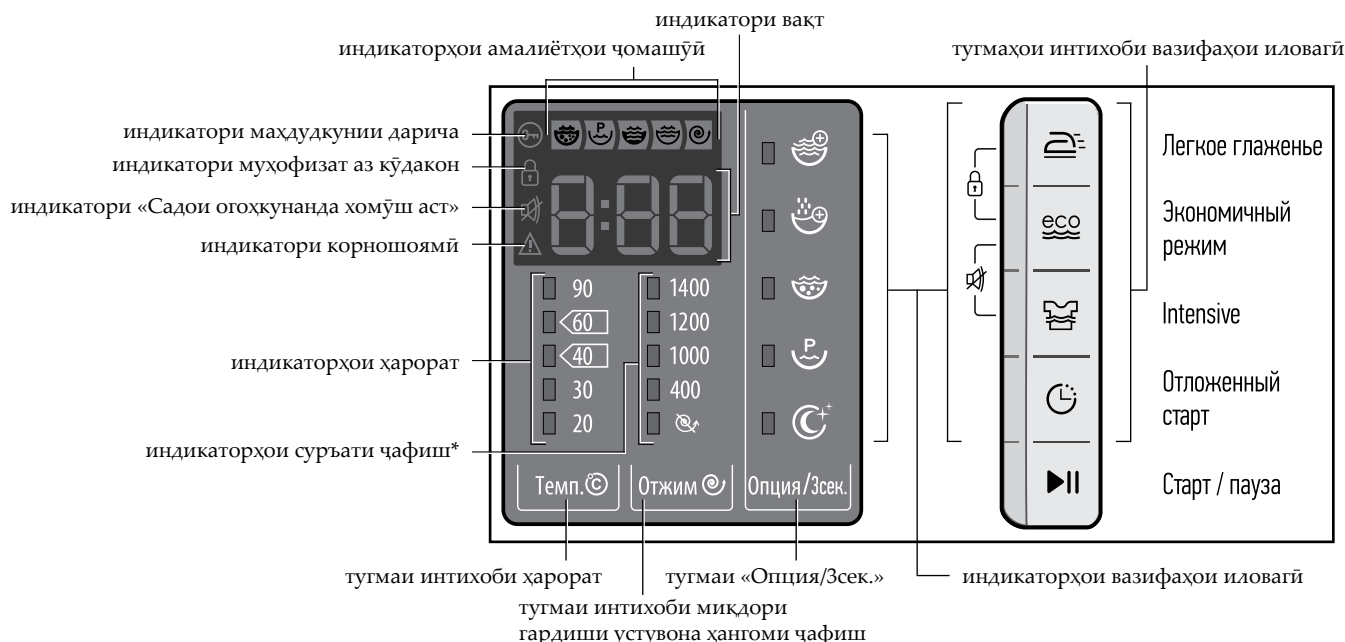
Расми 3 – Худуди индикаторҳо ва тутмаҳои идоракунӣ
