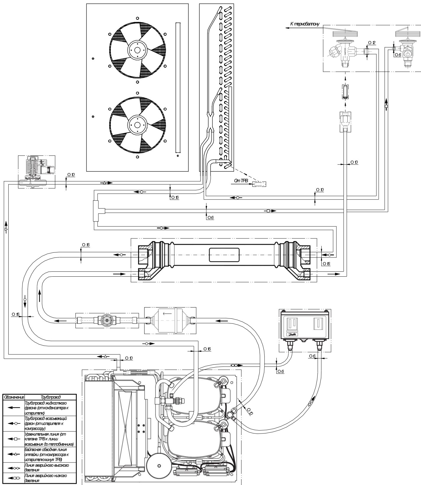
Функциональная схема системы охлаждения
