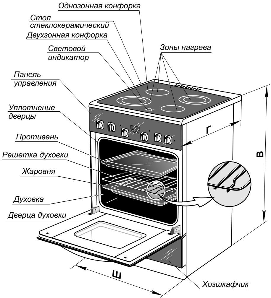
Рис. 2 Плита 6560, 5560, 6760, 5160
